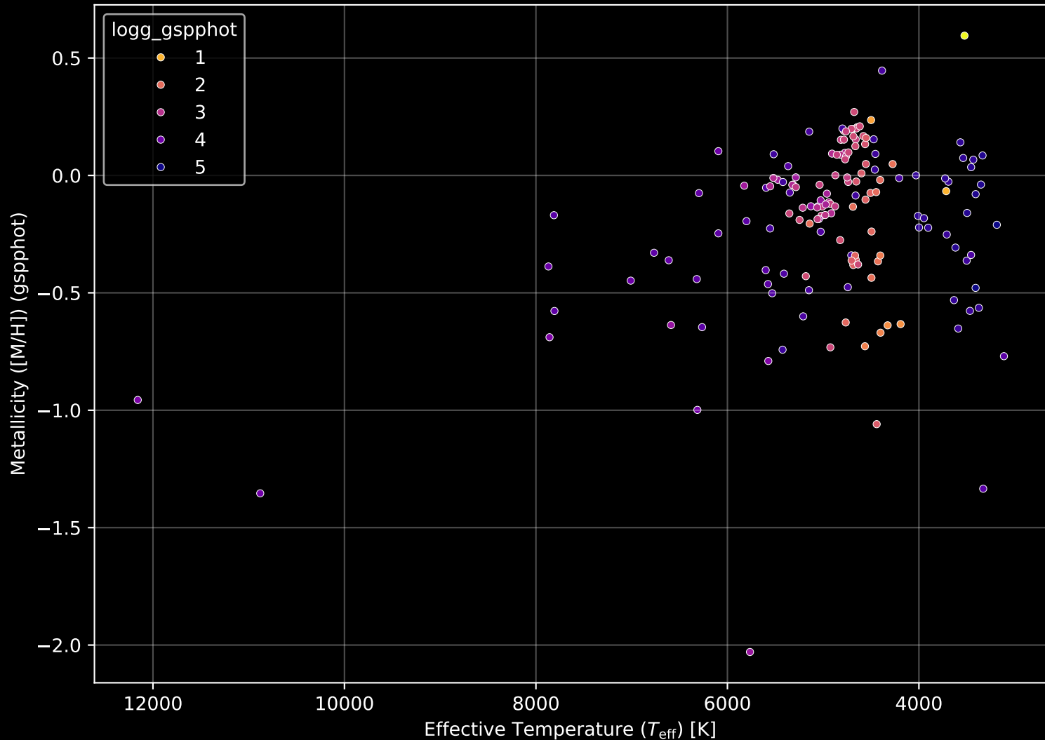
APOGEE DR17 Field: [K2_C7_012-17] Stellar Population Parameters (n= 154)
